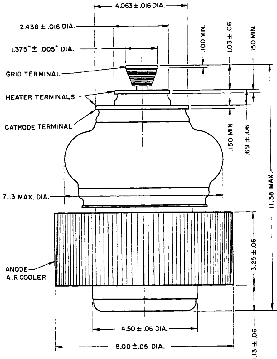
DIMENSIONS — ML-7003
